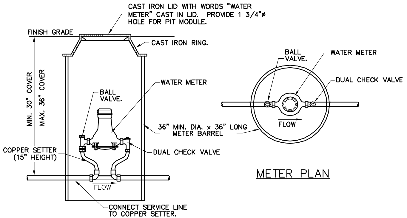
METER SECTION
