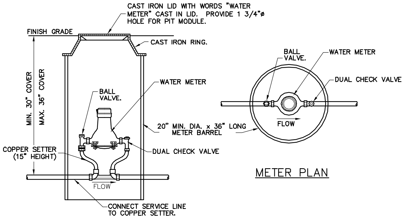
METER SECTION
